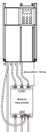
Рис. В-2 Установка простого фильтра ЭМС
