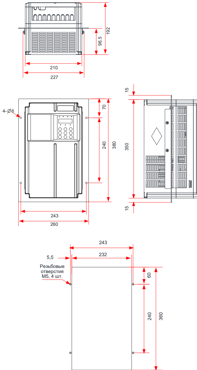
Рис. 9-8 Размеры монтажного кронштейна и расстояние между отверстиями для моделей инверторов мощностью 18,5 – 22 кВт
