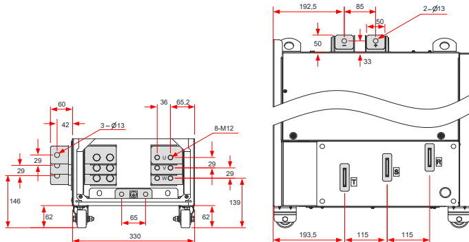
Рис. 3-49 Размеры клемм силовой цепи (CS710-4T250G/ CS710-4T280G, без моторного дросселя)
