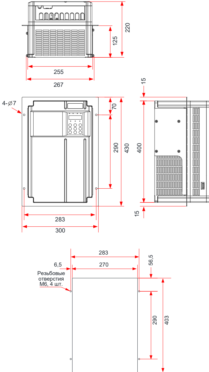
Рис. 9-9 Размеры монтажного кронштейна и расстояние между отверстиями для моделей инверторов мощностью 30 – 37 кВт
