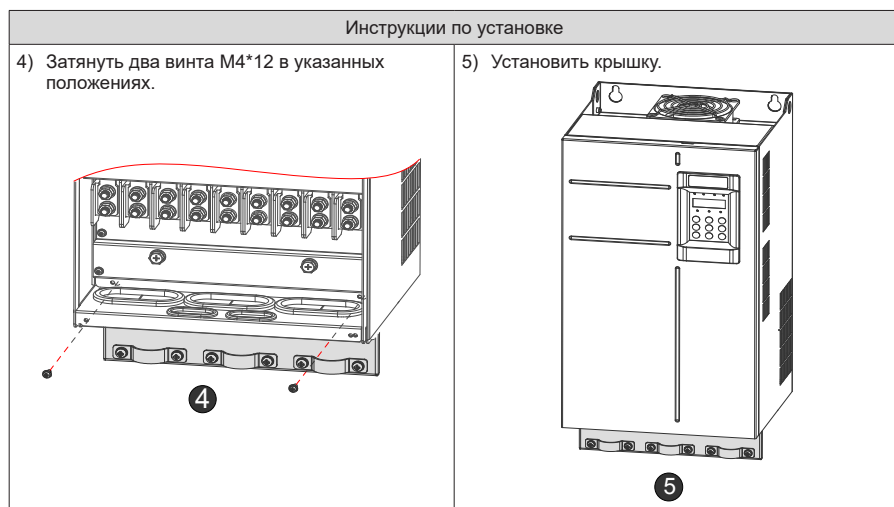
Рис. 3-34 Установка кронштейна заземления экранов кабеля
