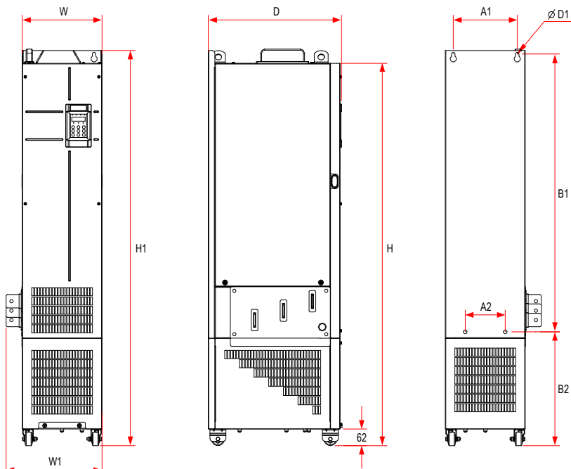
Рис. 9-14 Габаритные и монтажные размеры инверторов мощностью 200 – 450 кВт (с основанием под дроссель)
