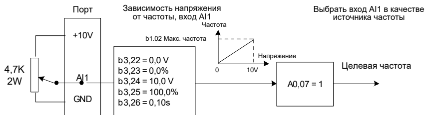
Рис. 5-7 Использование аналогового входа для установки задания частоты
