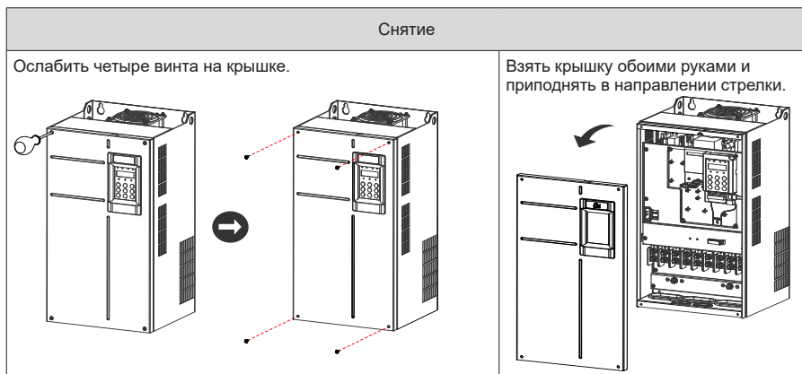
Рис. 3-23 Снятие и установка крышки моделей мощностью 0,4 – 37 кВт
