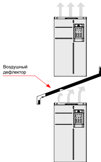
Рис. 3-5 Монтаж приводов в верхний и нижний ряды
