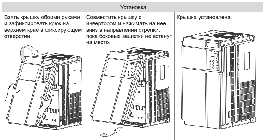
Рис. 3-23 Снятие и установка крышки моделей мощностью 0,4 – 37 кВт
