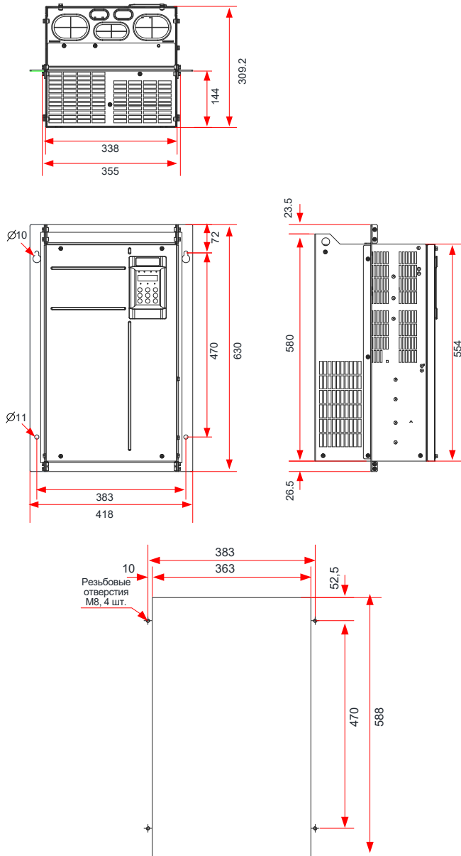
Рис. 9-11 Размеры монтажного кронштейна и расстояние между отверстиями для моделей инверторов мощностью 75 – 110 кВт
