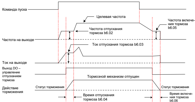
Рис. 5-9 Типовой процесс управления подъемной системой и настройка функции кода
