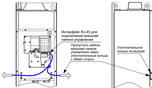
Рис. 3-70 Подключение внешней панели управления
