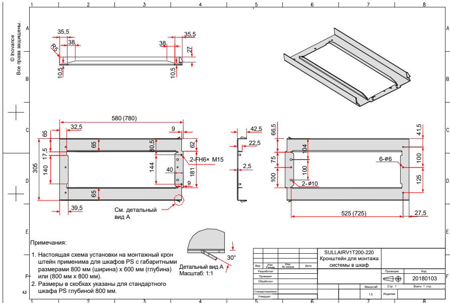
Рис. 9-15 Размеры монтажного кронштейна для моделей мощностью 200 – 220 кВт (стандартная конфигурация)
