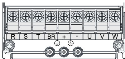
Рис. 3-27 Расположение клемм силовой цепи на инверторах мощностью 0,4 – 15 кВт
