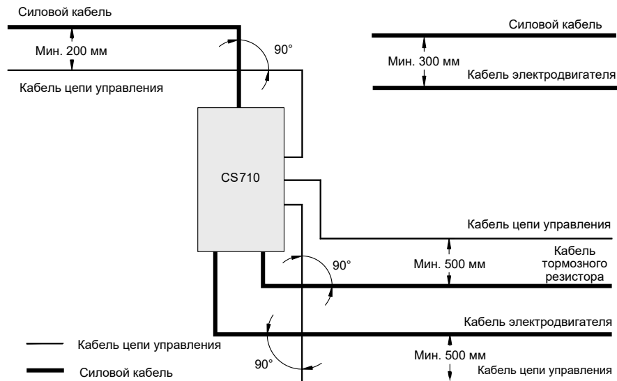
Рис. 3-58 Кабели
