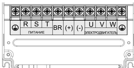
Рис. 3-28 Расположение клемм силовой цепи на инверторах мощностью 18,5 – 160 кВт
