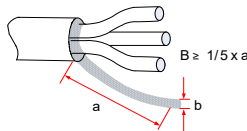
Рис. 3-35 Провод от экрана
