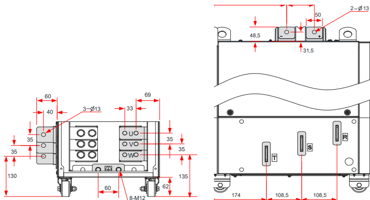
Рис. 3-46 Размеры клемм силовой цепи (CS710-4T200G/CS710-4T220G, без моторного дросселя)
