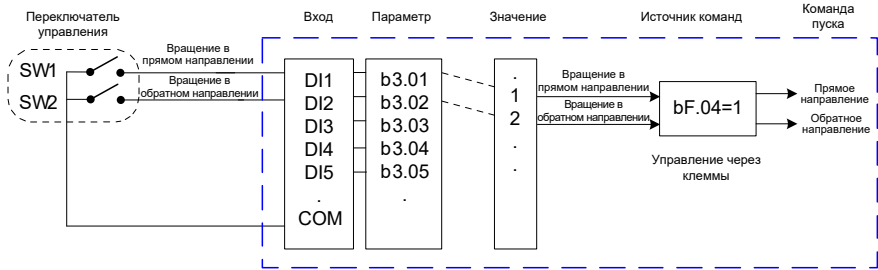
Рис. 5-2 Пример управления инвертором через клеммы
