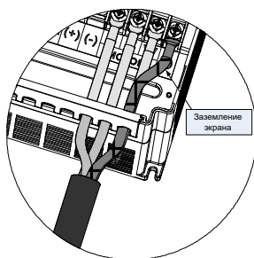
Рис. В-6 Заземление экранированного кабеля
