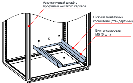
Рис. 3-17 Установка нижнего монтажного кронштейна
