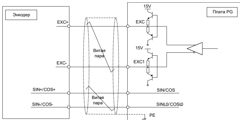
Рис. 10-11 Схема интерфейсов на плате MD38PG4
