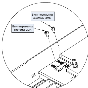
Рис. В-8 Винты-перемычки VDR и EMC
