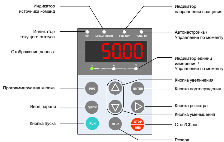
Рис. 4-1 Светодиодная панель управления
