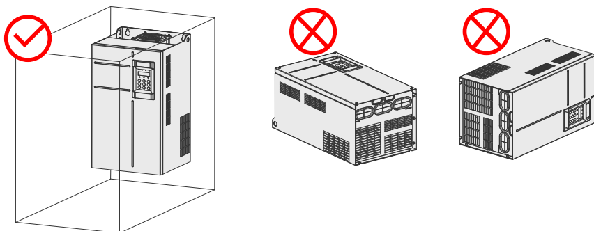
Рис. 3-6 Правильная и неправильная ориентация при монтаже
