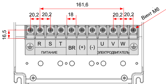
Рис. 3-42 Размеры клемм силовой цепи (CS710-4T30GB/CS710-4T37GB, три фазы 380 – 480 В)
