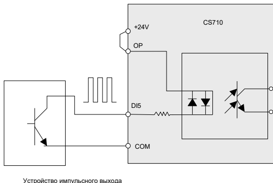
Рис. 3-65 Высокоскоростной импульсный вход
