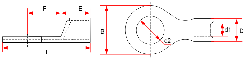
Рис. 9-18 Размеры наконечников серии TNR
