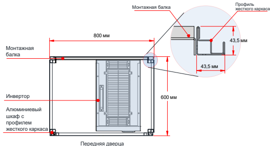
Рис. 3-15 Вид сверху шкафа 200 – 450 кВт
