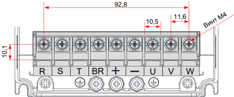
Рис. 3-38 Размеры клемм силовой цепи (CS710-4T0.4GB – CS710-4T5.5GB, три фазы 380 – 480 В)
