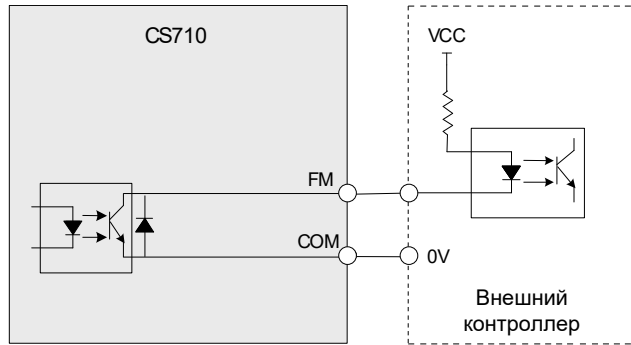
Рис. 3-67 Подключение высокоскоростного дискретного выхода FM
