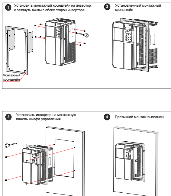
Рис. 3-9 Протычный монтаж для моделей мощностью 0,4 – 37 кВт
