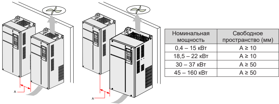
Рис. 3-4 Свободное пространство при параллельном монтаже группы инверторов
