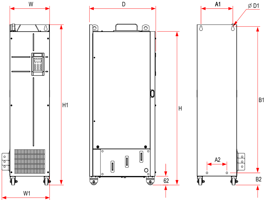
Рис. 9-13 Габаритные и монтажные размеры инверторов мощностью 200 – 450 кВт (без основания под дроссель)
