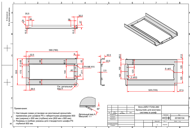
Рис. 9-16 Размеры монтажного кронштейна для моделей мощностью 250 – 280 кВт (стандартная конфигурация)
