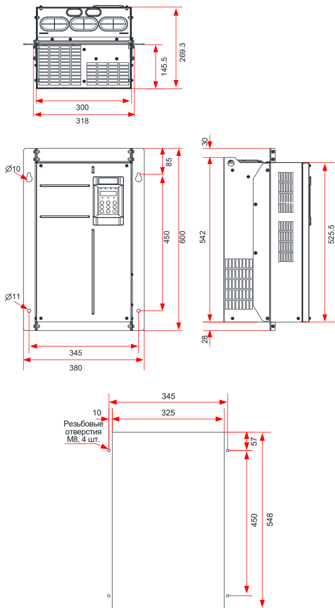
Рис. 9-10 Размеры монтажного кронштейна и расстояние между отверстиями для моделей инверторов мощностью 45 – 55 кВт
