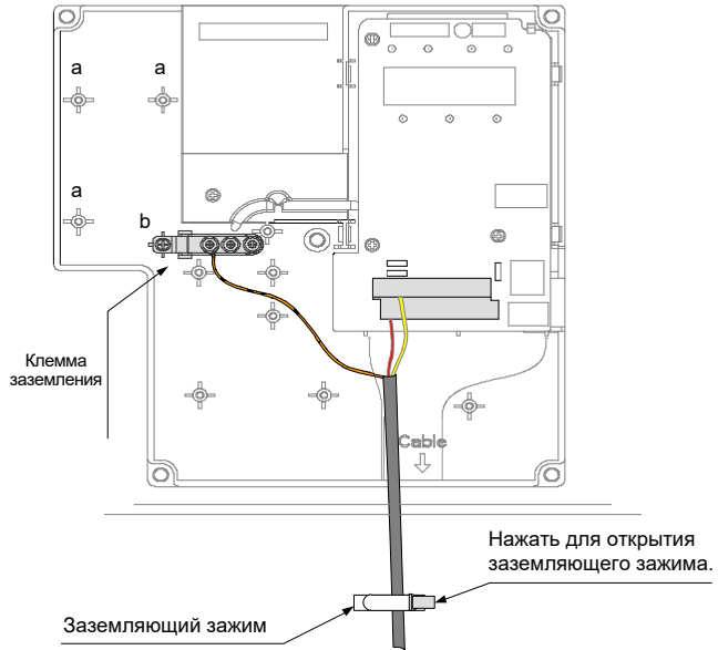
Рис. 3-60 Подключение экрана к клемме PE инвертора
