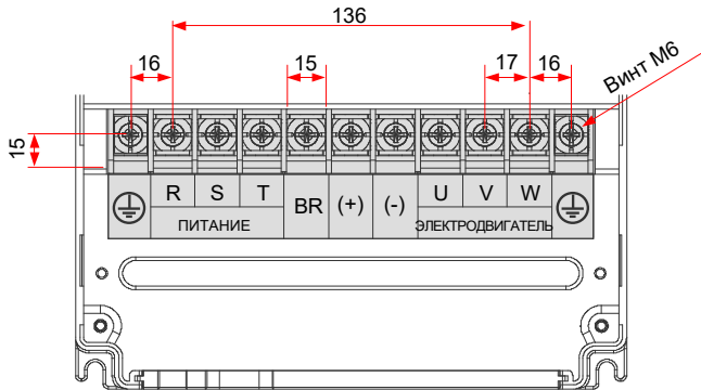
Рис. 3-41 Размеры клемм силовой цепи (CS710-4T18.5GB(-T)/ CS710-4T22GB(-T), три фазы 380 – 480 В)
