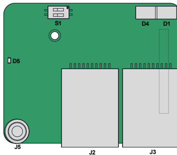
Рис. 10-10 Расположение клемм на плате MD500-PN1
