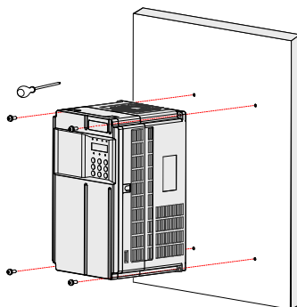
Рис. 3-7 Установка на монтажную панель для моделей мощностью 0,4 – 37 кВт
