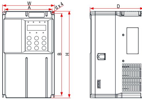
Рис. 9-1 Габаритные и монтажные размеры моделей инверторов мощностью 0,4 – 15 кВт
