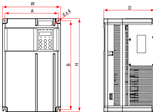
Рис. 9-2 Габаритные и монтажные размеры моделей инверторов мощностью 18,5 – 37 кВт
