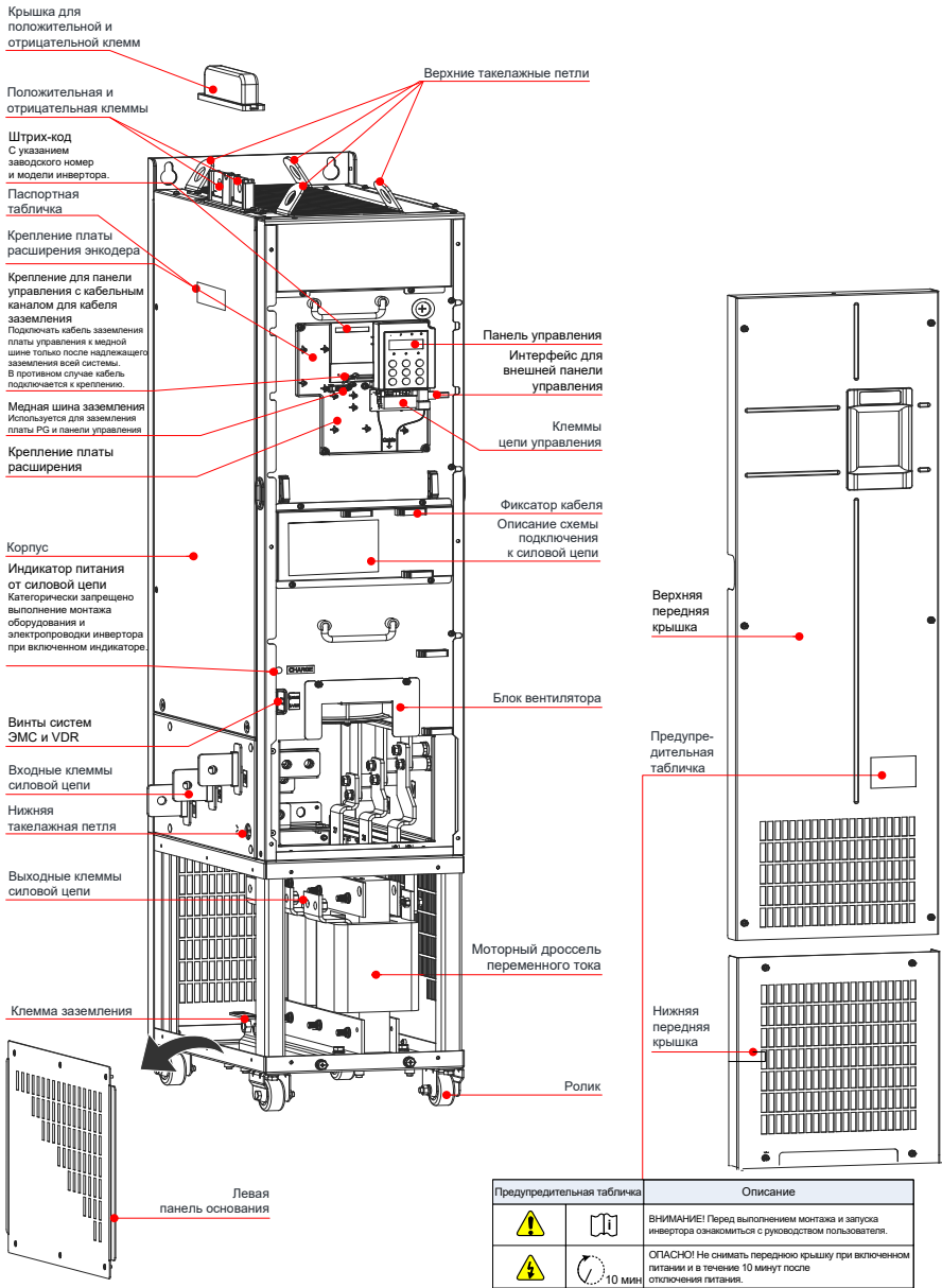
Рис. 1-6 Комплектующие (три фазы 380 – 480 В, 200 – 450 кВт (-L))
