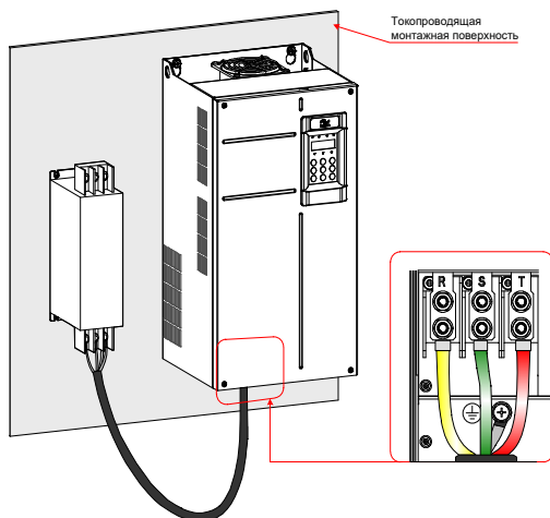
Рис. 3-32 Монтаж фильтра
