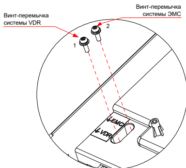
Рис. 3-37 Винт VDR и винт EMC
