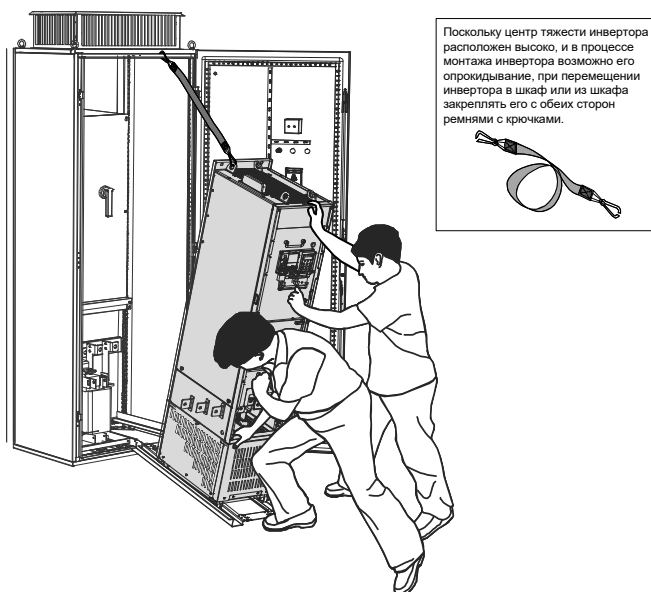
Рис. 3-20 Вставка инвертора в шкаф
