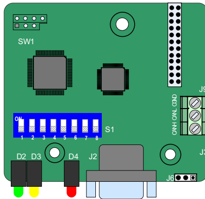
Рис. 10-9 Схема расположения клемм на плате MD38DP2
