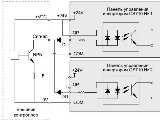
Рис. 3-63 Параллельное соединение дискретных входов (DI) нескольких инверторов в режиме ПРИЕМНИКА (SINK)
