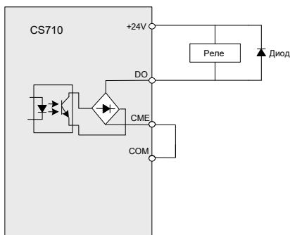
Рис. 3-66 Подключение дискретного выхода (DO)
