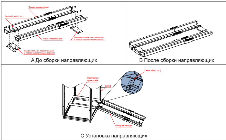
Рис. 3-18 Установка направляющих в шкаф
