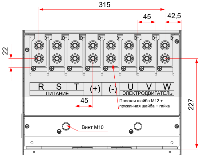
Рис. 3-45 Размеры клемм силовой цепи (CS710-4T132G/CS710-4T160G)
