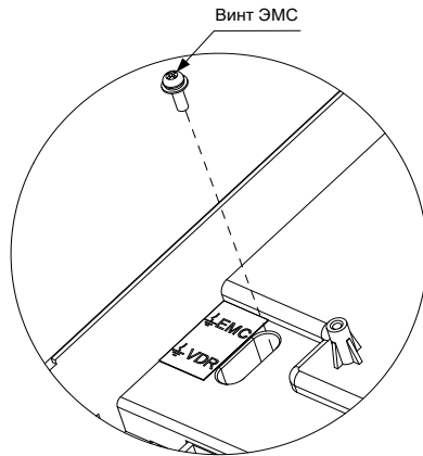
Рис. 9-21 Отсоединение винта EMC
