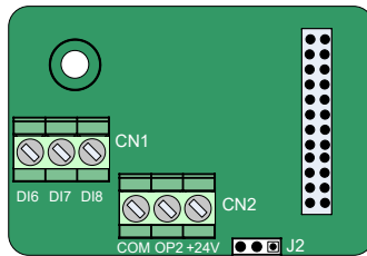
Рис. 10-2 Схема расположения клемм на плате MD38IO2
