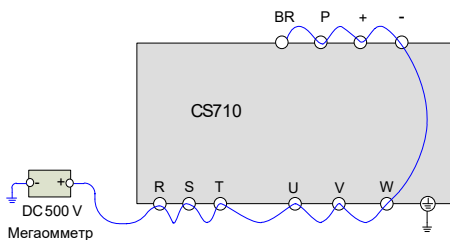
Рис. 8-1 Испытание изоляции силовой цепи
