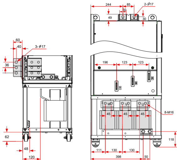
Рис. 3-53 Размеры клемм силовой цепи (CS710-4T315G-L – CS710-4T450G-L, с моторным дросселем)
