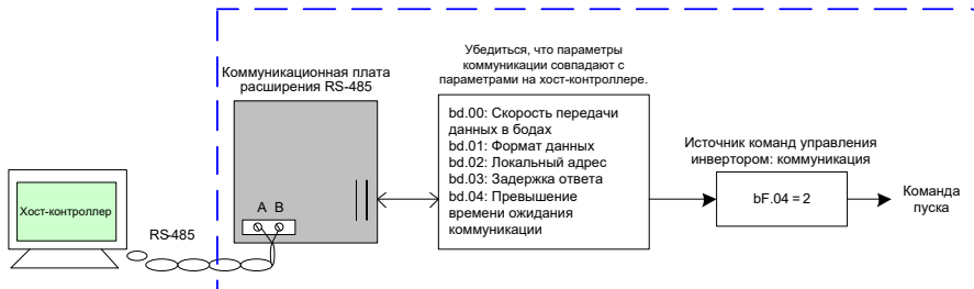
Рис. 5-3 Пример управления инвертором посредством коммуникации с хост-контроллером
