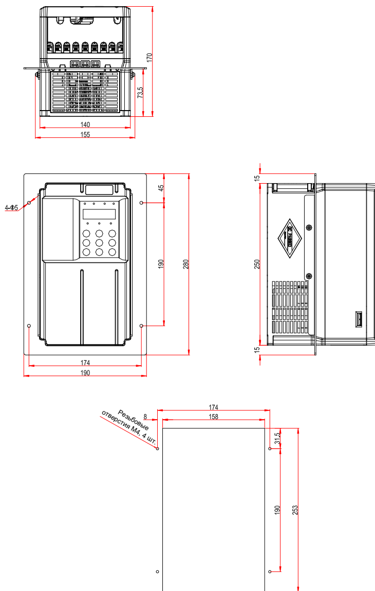
Рис. 9-6 Размеры монтажного кронштейна и расстояние между отверстиями для моделей инверторов мощностью 7,5 – 11 кВт
