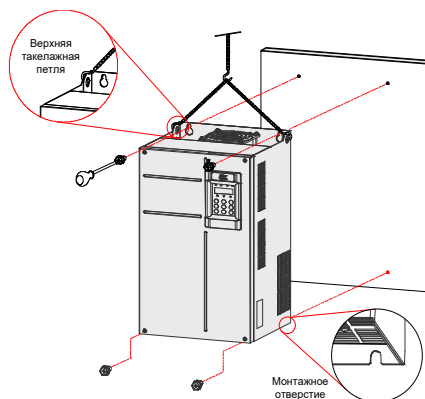
Рис. 3-8 Установка на монтажную панель для моделей мощностью 45 – 160 кВт
