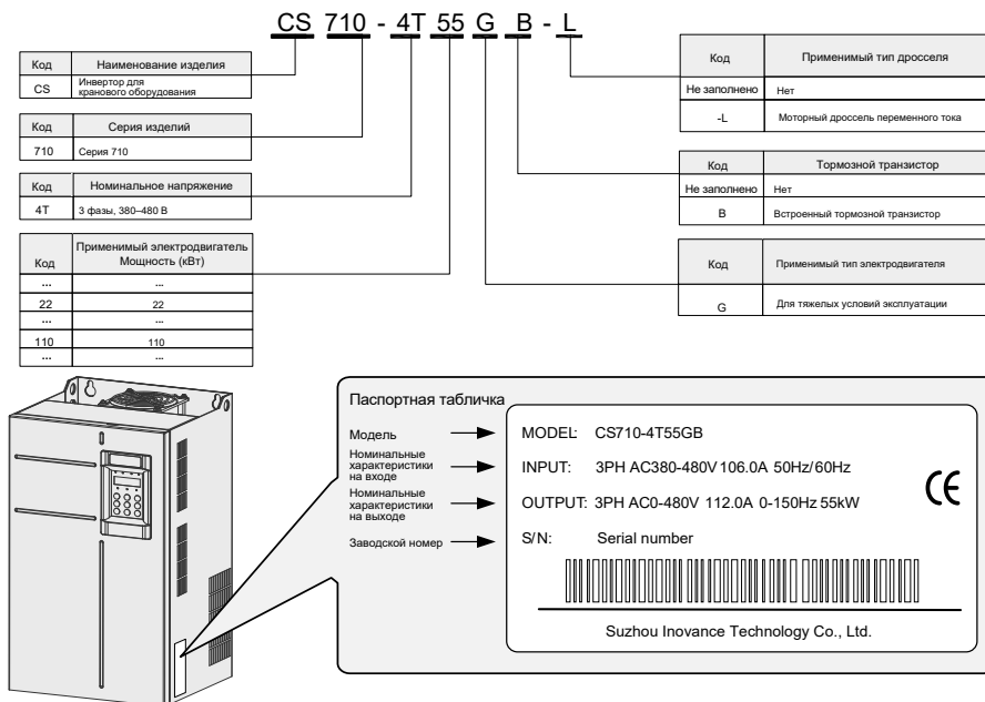
Рис. 1-1 Заводская табличка и номер модели
