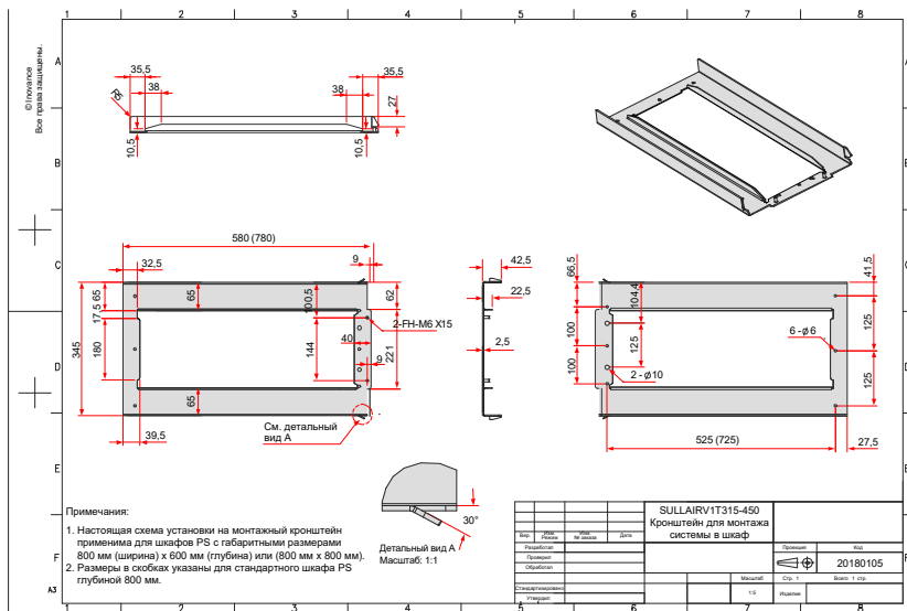
Рис. 9-17 Размеры монтажного кронштейна для моделей мощностью 315 – 450 кВт (стандартная конфигурация)
