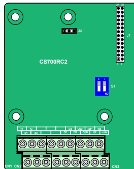
Рис. 10-5 Схема расположения клемм на плате CS700RC2
