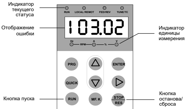
Рис. 7-2 Светодиодная индикация ошибки
