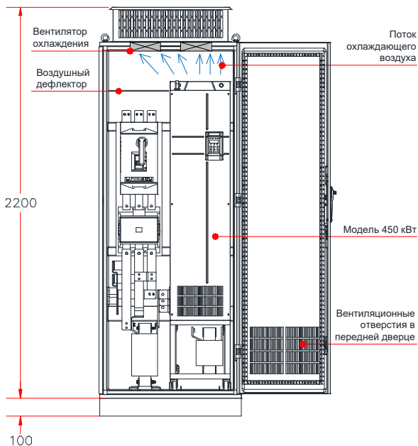
Рис. 3-12 Шкаф с принудительной вентиляцией
