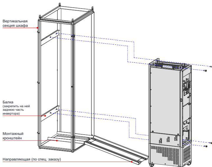
Рис. 3-22 Крепление инвертора к балкам на задней стороне части шкафа через четыре монтажных отверстия на задней стороне инвертора.
