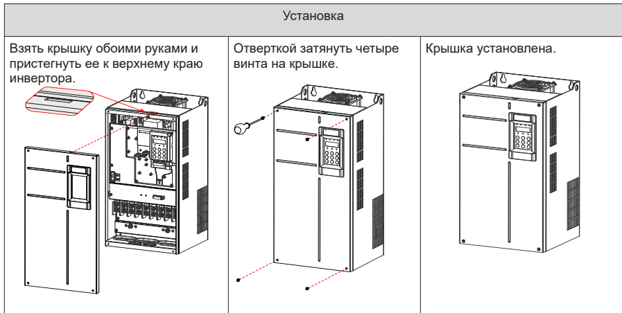
Рис. 3-24 Снятие и установка крышки моделей мощностью 45 – 160 кВт
