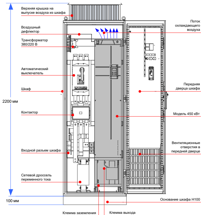
Рис. 3-14 Рекомендуемая компоновка шкафа
