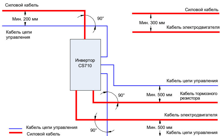
Рис. В-7 Схема подключения кабелей
