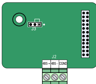
Рис. 10-8 Схема расположения клемм на плате MD38TX1
