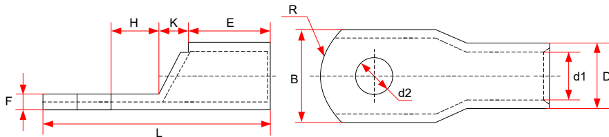
Рис. 9-19 Размеры наконечников серии GTNR
