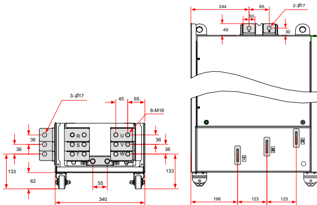
Рис. 3-52 Размеры клемм силовой цепи (CS710-4T315G – CS710-4T450G, без моторного дросселя)
