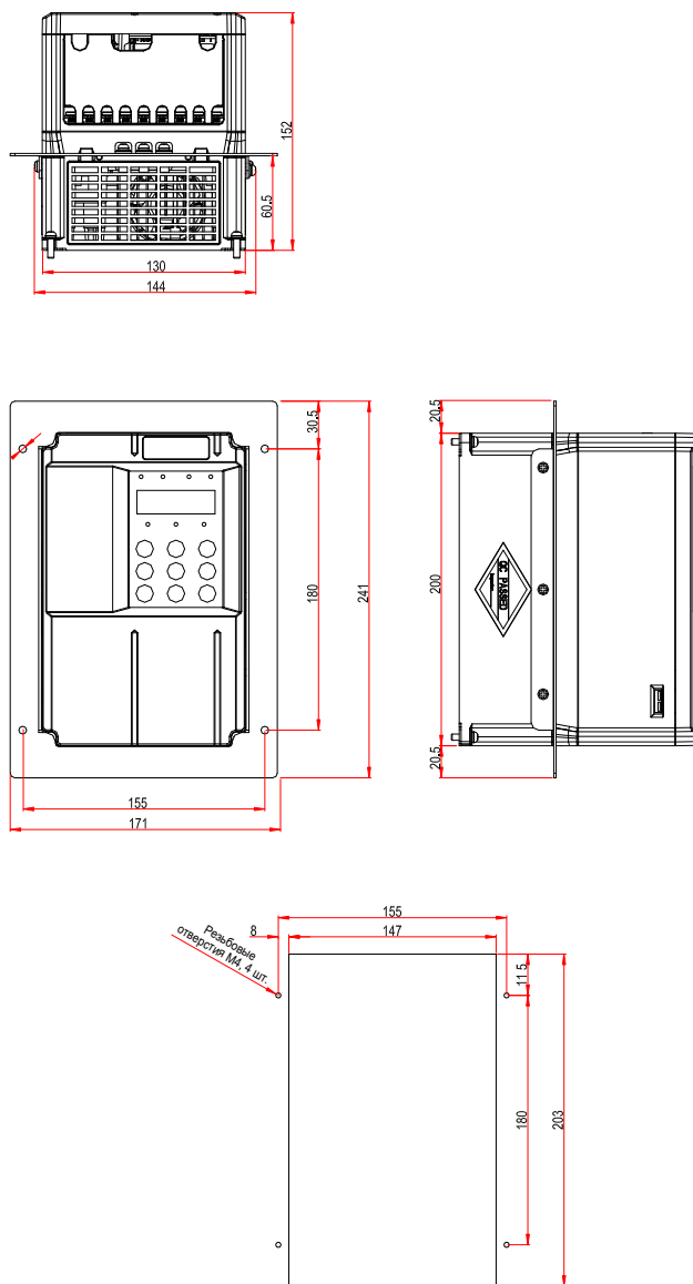
Рис. 9-4 Размеры монтажного кронштейна и расстояние между отверстиями для моделей инверторов мощностью 0,4 – 3,0 кВт
