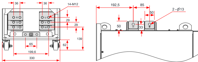
Рис. 3-51 Размеры клемм главной цепи (CS710-4T250G/CS710-4T280G, без медной шины с боковым вводом и моторного дросселя)
