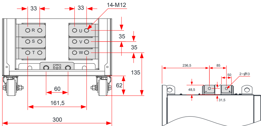
Рис. 3-48 Размеры клемм главной цепи (CS710-4T200G-L/CS710-4T220G-L, без медной шины с боковым вводом и моторного дросселя)
