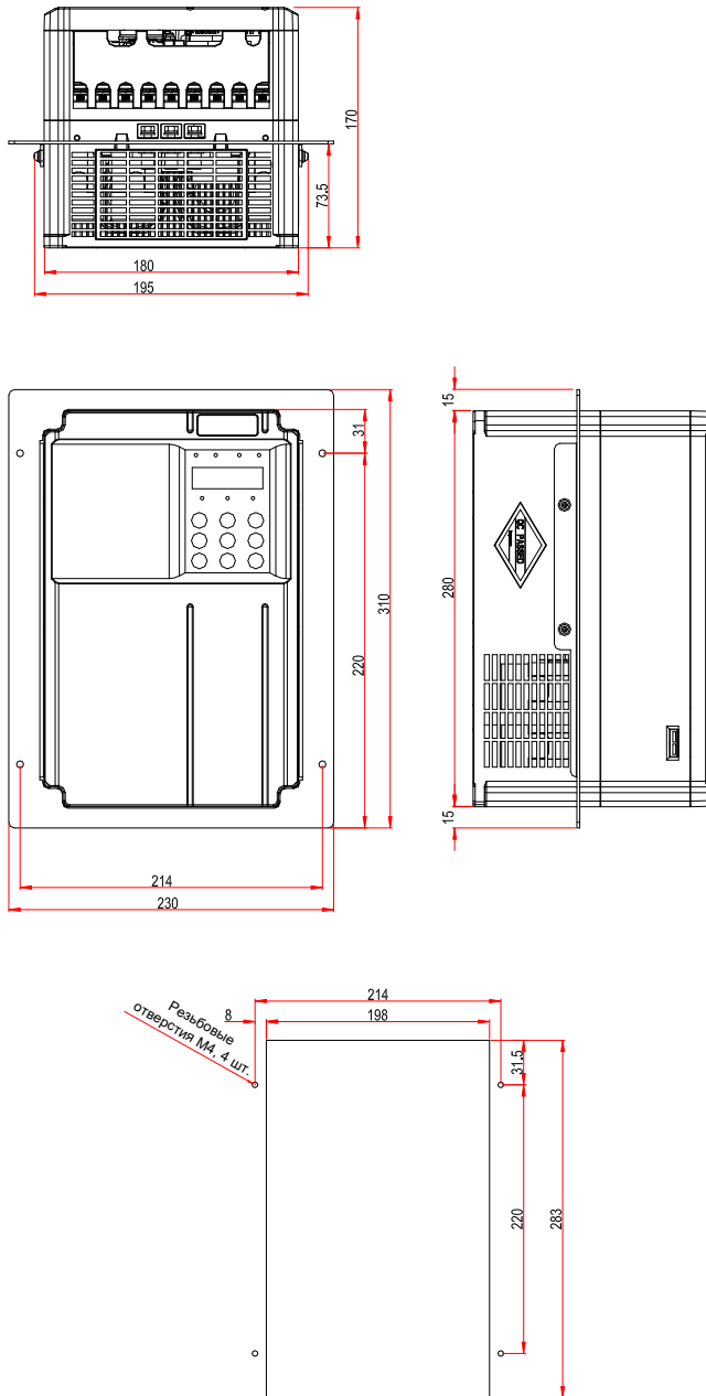
Рис. 9-7 Размеры монтажного кронштейна и расстояние между отверстиями для моделей инверторов мощностью 15 кВт
