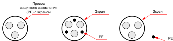
Рис. 3-30 Рекомендуемые силовые кабели
