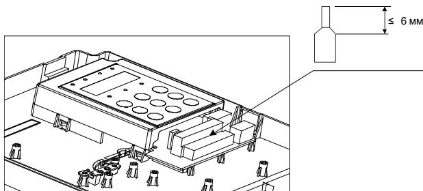
Рис. 3-69 Размеры наконечника
