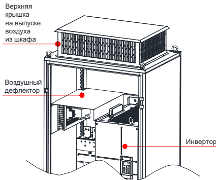
Рис. 3-13 Изолирующий барьер в шкафу
