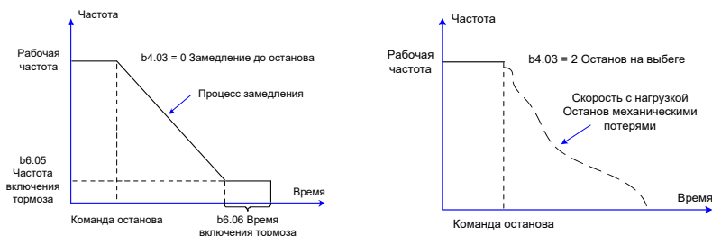
Рис. 5-4 Режимы останова
