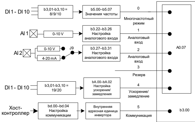
Рис. 5-5 Выбор источника задания частоты
