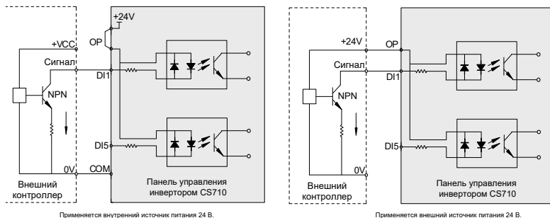
Рис. 3-62 Подключение ПРИЕМНИКА
