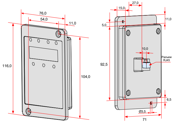
Рис. 9-23 Размеры MD32NKE1 (мм)
