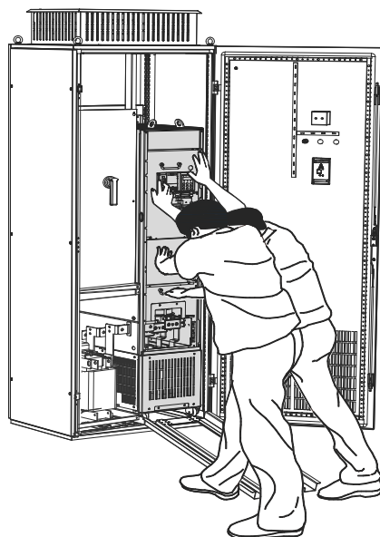
Рис. 3-21 Инвертор, вставленный в шкаф
