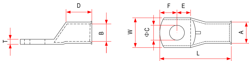
Рис. 9-20 Размеры наконечников серии BC
