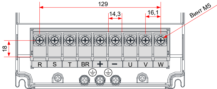
Рис. 3-40 Размеры клемм силовой цепи (CS710-4T15GB, три фазы 380 – 480 В)
