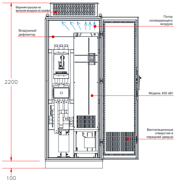
Рис. 3-11 Самовентилируемый шкаф
