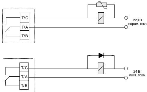
Рис. 3-68 Подключение релейной клеммы
