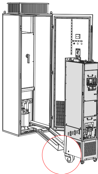
Рис. 3-19 Выравнивание роликов инвертора относительно направляющих
