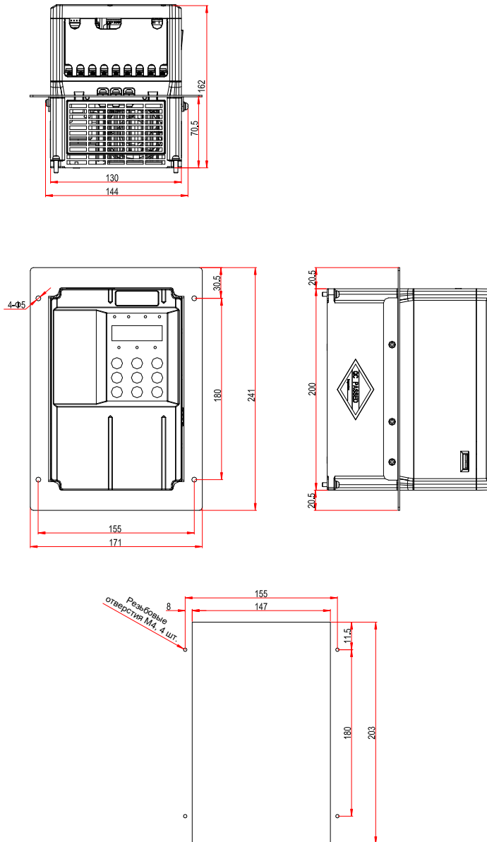
Рис. 9-5 Размеры монтажного кронштейна и расстояние между отверстиями для моделей инверторов мощностью 3,7 – 5,5 кВт
