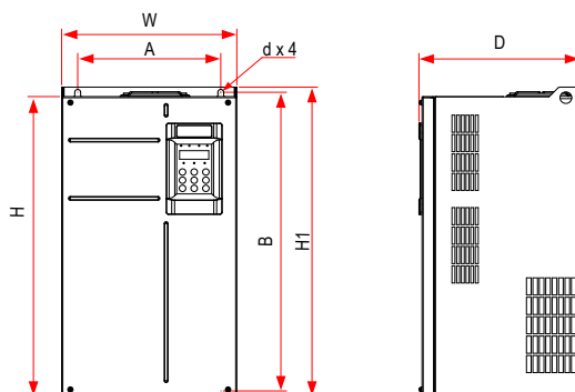
Рис. 9-3 Габаритные и монтажные размеры моделей инверторов мощностью 45 – 160 кВт
