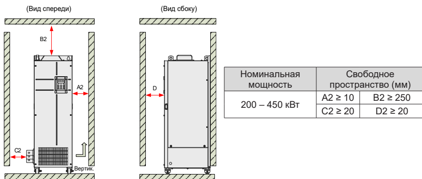
Рис. 3-3 Свободное пространство при монтаже одиночного инвертора (три фазы 380 – 480 В 200 э 450 кВт)
