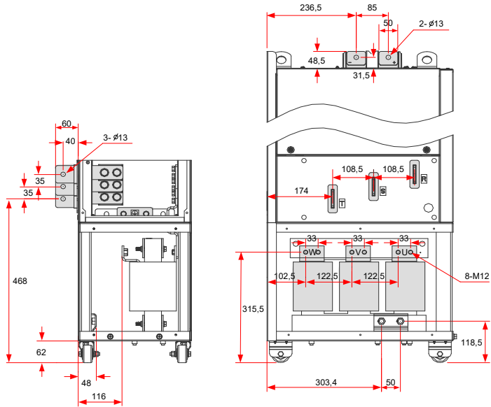
Рис. 3-47 Размеры клемм силовой цепи (CS710-4T200G-L/CS710-4T220G-L, с моторным дросселем)
