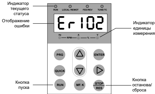
Рис. 7-1 Отображение ошибки
