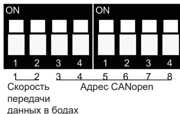
Рис. 10-7 DIP-переключатели MD38CAN2
