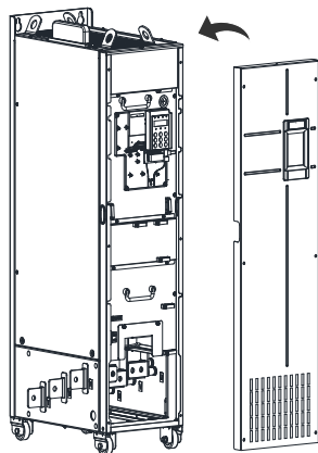
Рис. 3-25 Снятие и установка крышки моделей мощностью 200 – 450 кВт
