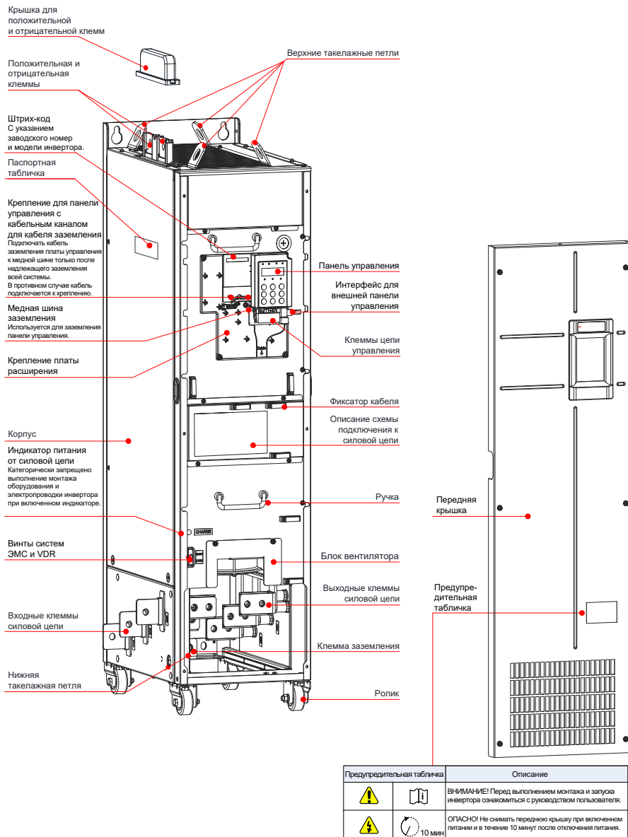
Рис. 1-5 Комплектующие (три фазы 380 – 480 В, 200 – 450 кВт)
