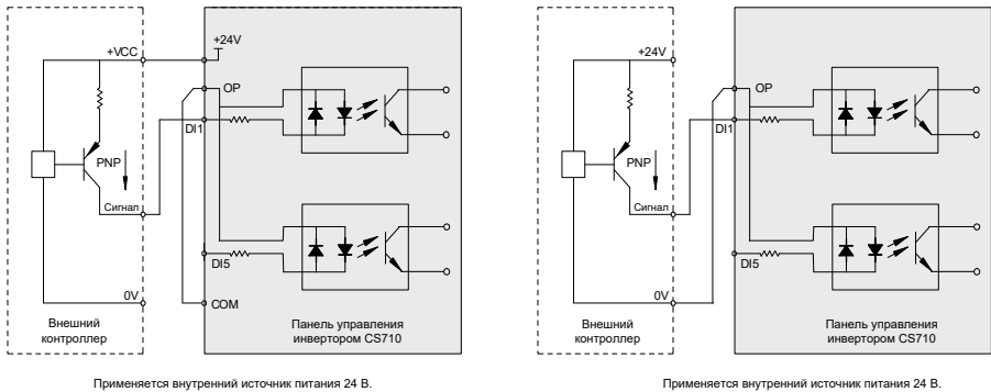
Рис. 3-64 Подключение в режиме ИСТОЧНИКА (SOURCE)
