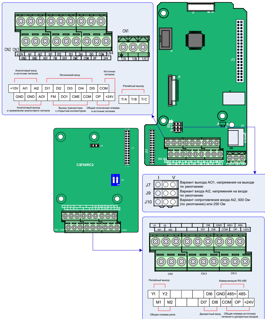
Рис. 3-56 Расположение клемм цепи управления
