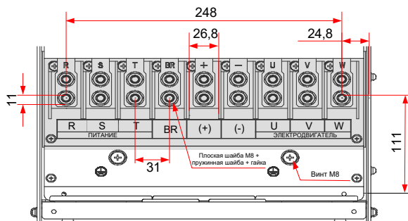
Рис. 3-43 Размеры клемм силовой цепи (CS710-4T45GB/ CS710-4T55GB, три фазы 380 – 480 В)
