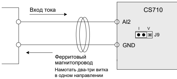
Рис. 3-61 Подключение AI2
