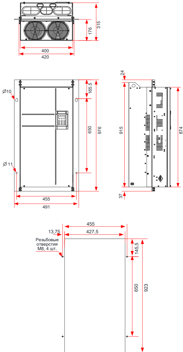
Рис. 9-12 Размеры монтажного кронштейна и расстояние между отверстиями для моделей инверторов мощностью 132 – 160 кВт
