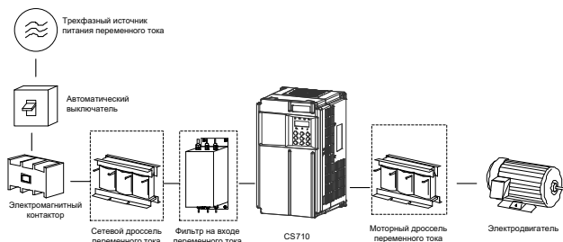
Рис. В-1 Монтаж периферийных устройств ЭМС (в границах пунктирных линий)
