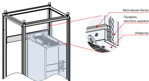
Рис. 3-16 Изометрический вид шкафа 200–450 кВт
