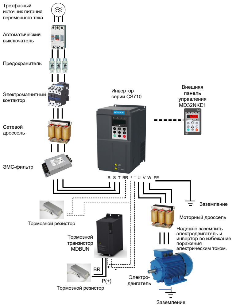
Рис. 2-1 Состав системы инвертора серии CS710
