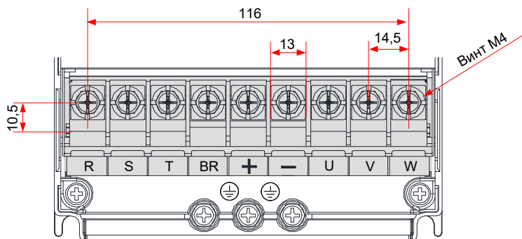
Рис. 3-39 Размеры клемм силовой цепи (CS710-4T7.5GB/CS710-4T11GB, три фазы 380 – 480 В)
