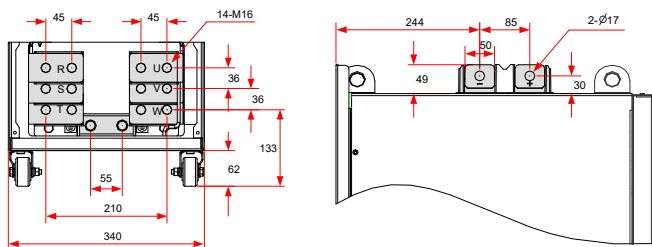
Рис. 3-54 Размеры клемм главной цепи (CS710-4T315G – CS710-4T450G, без медной шины с боковым вводом и моторного дросселя)
