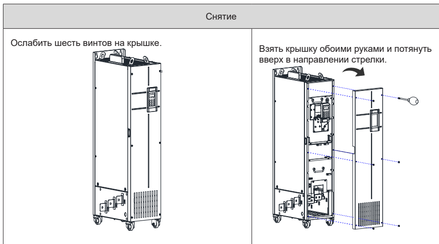
Рис. 3-24 Снятие и установка крышки моделей мощностью 45 – 160 кВт
