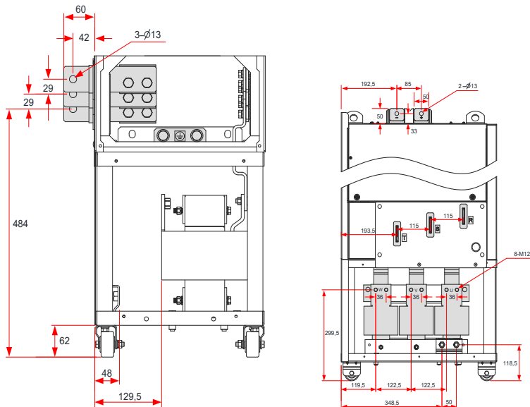
Рис. 3-50 Размеры клемм силовой цепи (CS710-4T250G-L/ CS710-4T280G-L, с моторным дросселем)
