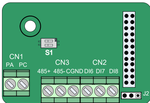
Рис. 10-3 Схема расположения клемм на плате MD38IO3
