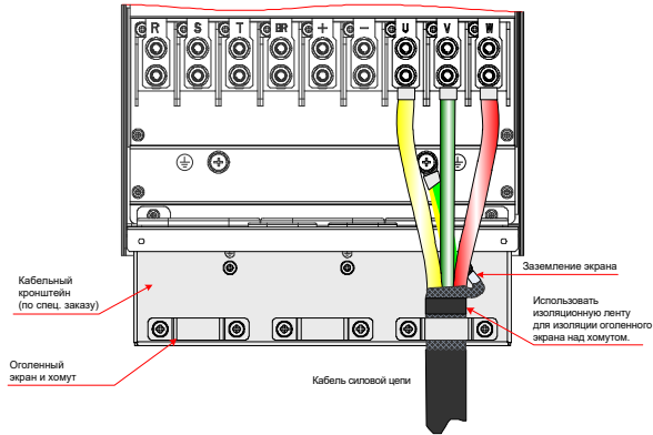
Рис. 3-33 Подключение экрана
