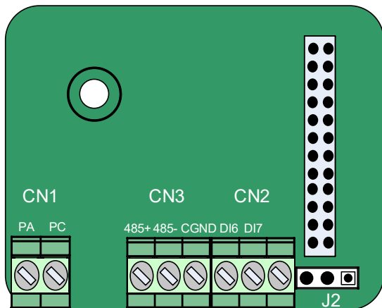
Рис. 10-4 Схема расположения клемм на плате CS700IO1
