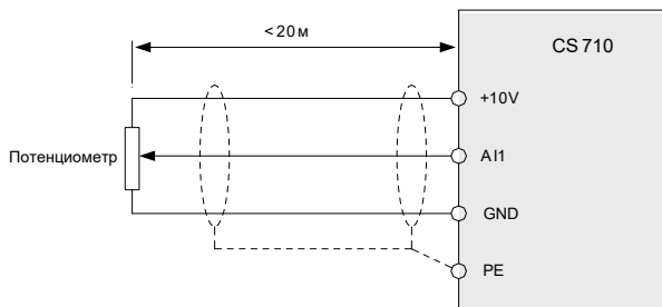
Рис. 3-59 Подключение A11
