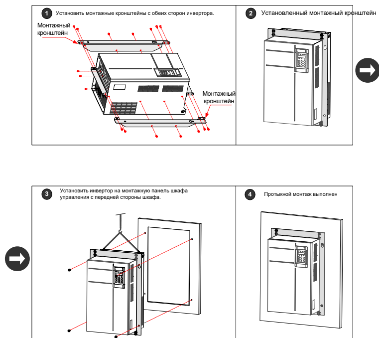
Рис. 3-10 Протычный монтаж для моделей мощностью 45 – 160 кВт
