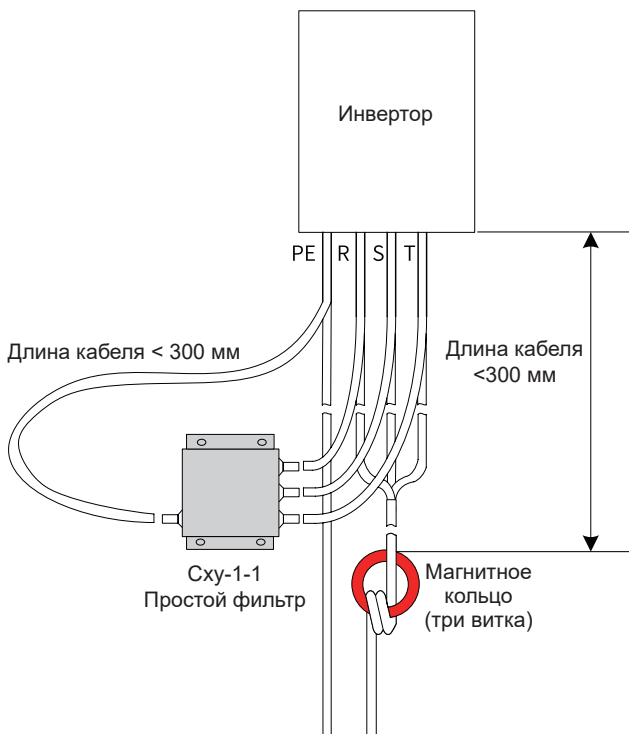
Рис. 9-22 Установка простого фильтра и магнитного кольца на входе
