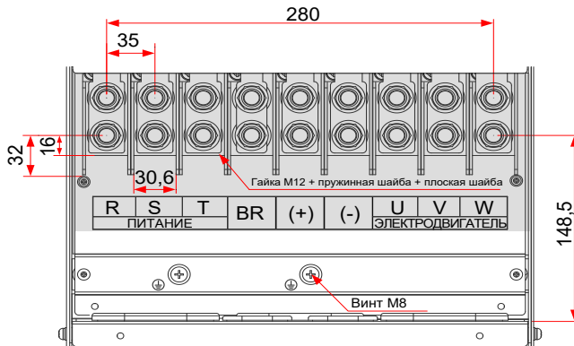
Рис. 3-44 Размеры клемм силовой цепи (CS710-4T75GB – CS710-4T110G, три фазы 380 – 480 В)
