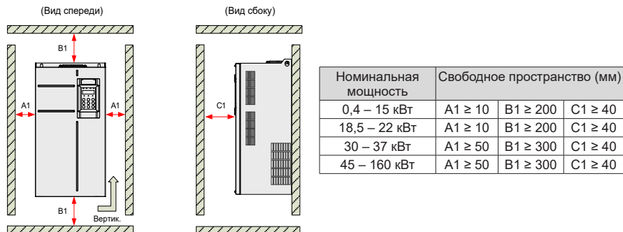
Рис. 3-2 Свободное пространство при монтаже одиночного инвертора (три фазы 380 – 480 В, 0,4 – 160 кВт)
