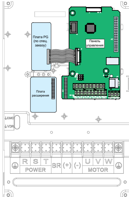
Рис. 3-55 Монтажное положение панели управления инвертора CS710
