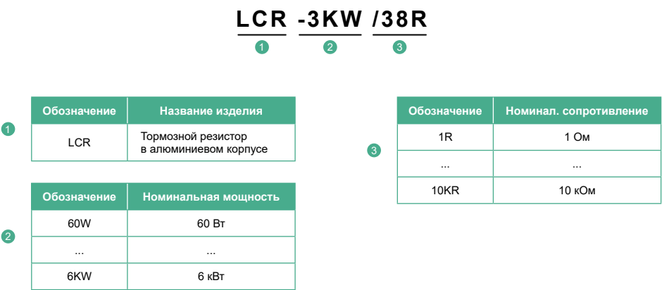
Рисунок 1.1 – Маркировка тормозного резистора LCR
